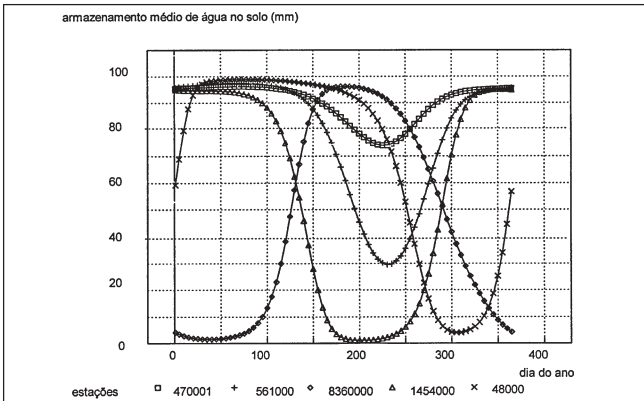
Figura 23. Armazenamento médio de água no solo (mm), para cada dia do ano, para estações representativas das áreas noroeste (470001), centro (561000), norte (8630000), sul (1454000) e leste (48000).
