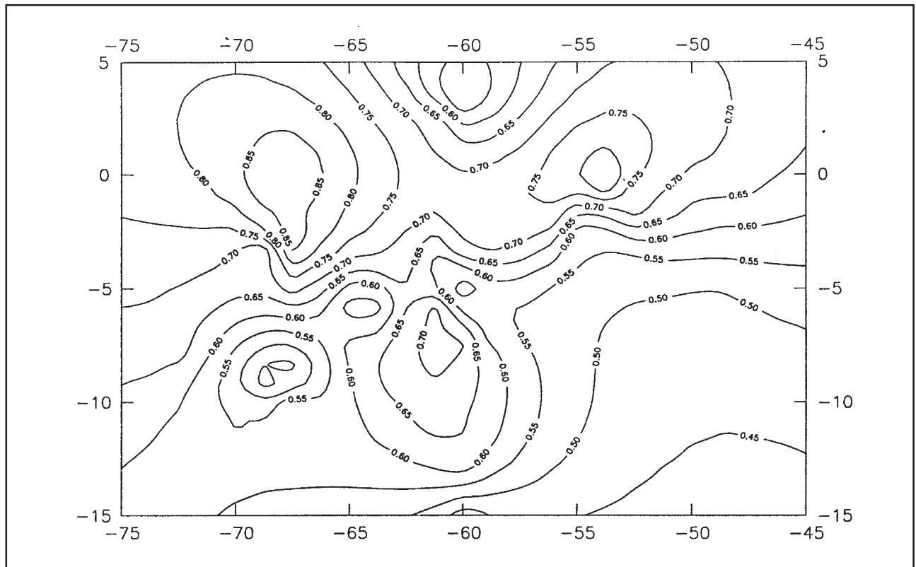
Figura 9. Probabilidade média anual de ocorrer 3 dias úmidos, em intervalos de 15 dias.
