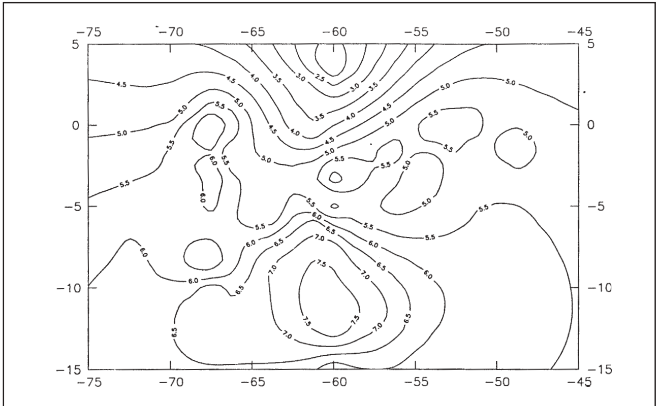
Figura 3. Número de dias chuvosos, num período de 10 dias, iniciando em 1º/01.
