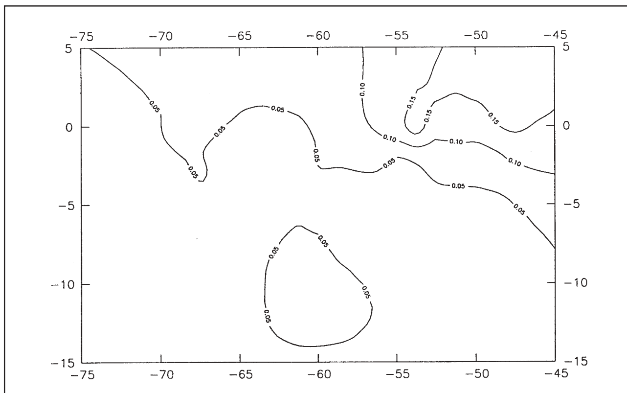
Figura 11. Probabilidade média anual de ocorrer 10 dias úmidos, em intervalos de 15 dias.
