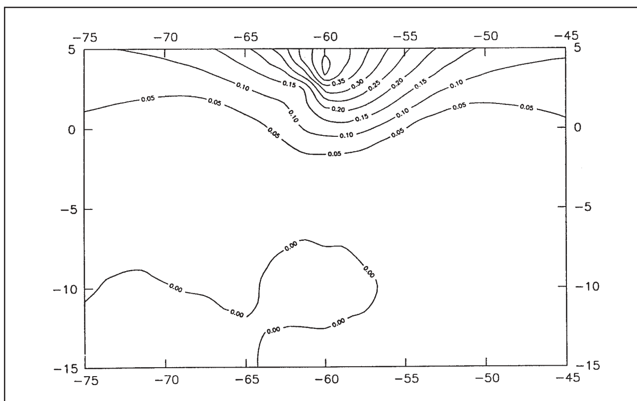
Figura 12. Probabilidade de ocorrer 10 dias secos, num intervalo de 15 dias, iniciando em 1º/01.
