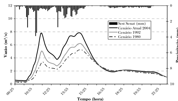
Figura 16 – Hidrogramas do evento do dia 09/11/2004
