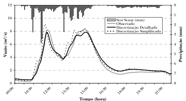
Figura 12 – Hidrograma obtido para a discretização detalhada e simplificada, para o evento do dia 09/11/04
