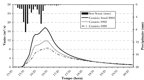
Figura 13 – Hidrogramas do evento do dia 10/06/2004
