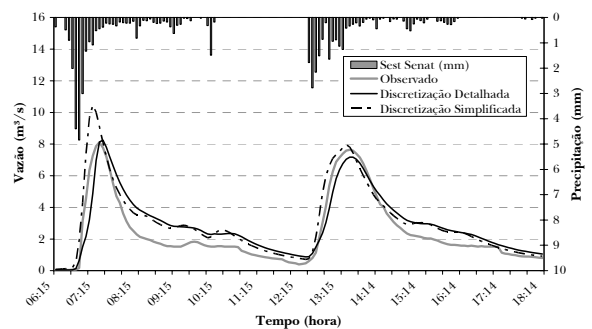
Figura 11 – Hidrograma obtido para a discretização detalhada e simplificada, para o evento do dia 16/10/04
