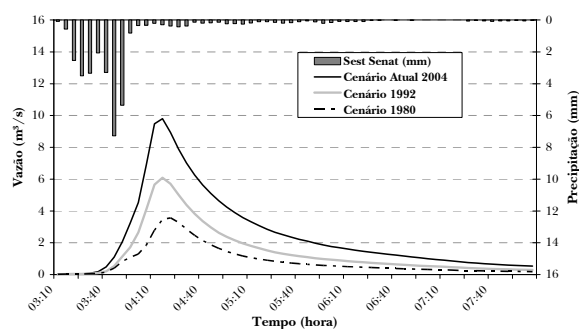
Figura 17 – Hidrogramas do evento do dia 06/12/2004
