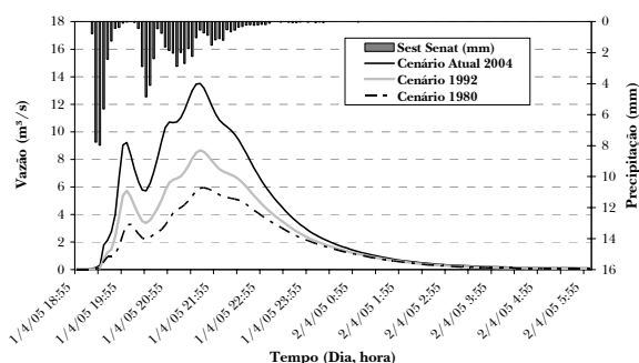
Figura 18 – Hidrogramas do evento do dia 01/04/2005
