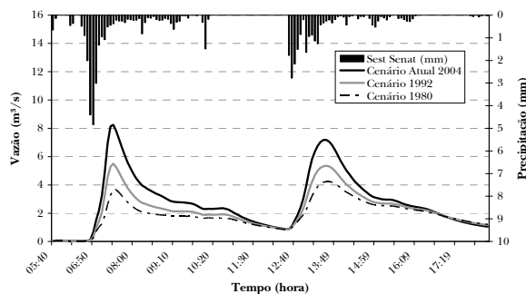
Figura 14 – Hidrogramas do evento do dia 16/10/2004
