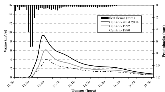
Figura 15 – Hidrogramas do evento do dia 03/11/2004
